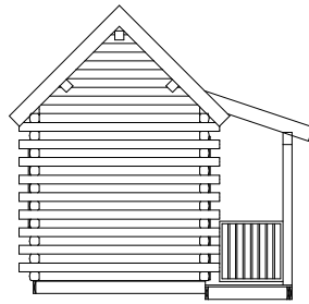
LEFT
